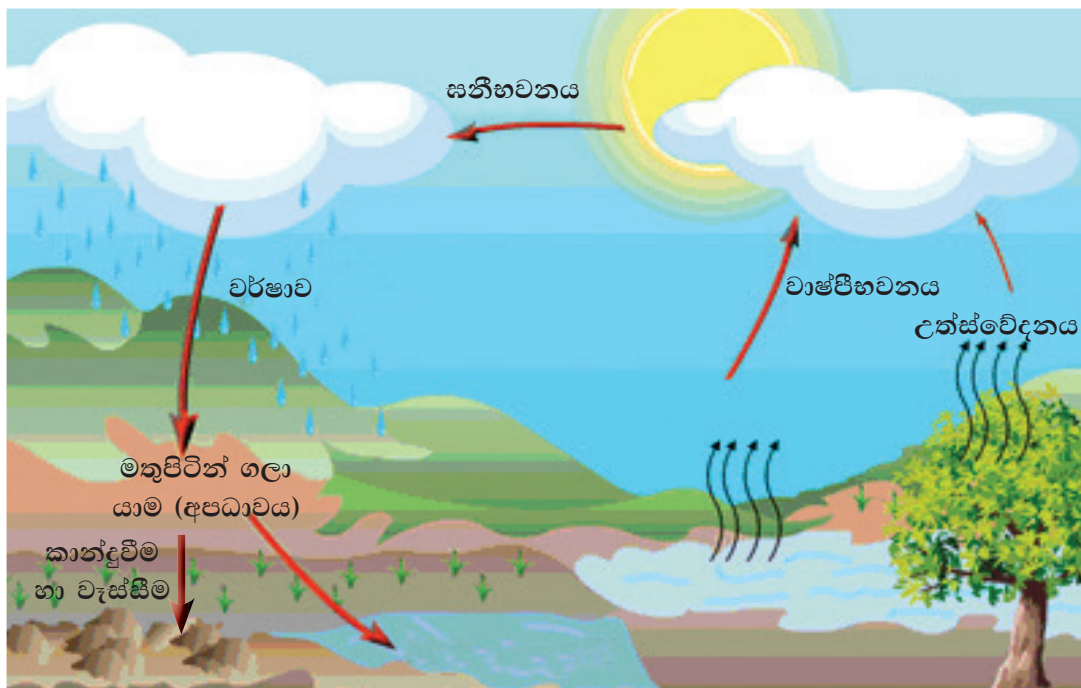
3.43 රූපය - ජල චක්‍රය
