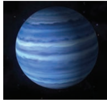
2.12 රූපය - නෙප්චූන්
