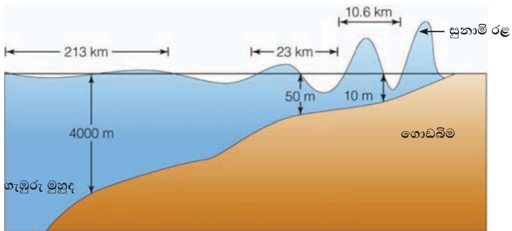
6.21 රූපය - සුනාමියක දී ජල තරංග ඇතිවන අයුරු
