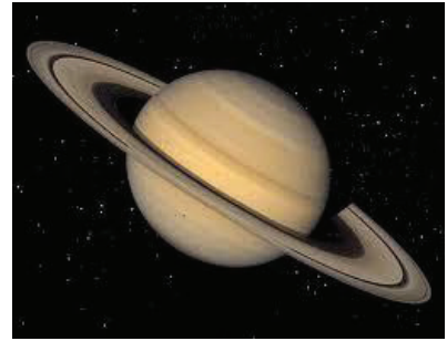
2.10 රූපය - සෙනසුරු
