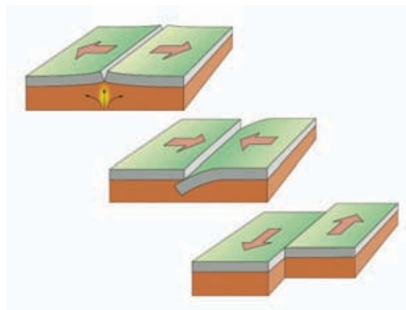
6.20 රූපය - භූ තැටි චලන ආකාර
