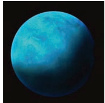
2.11 රූපය - යුරේනස්
