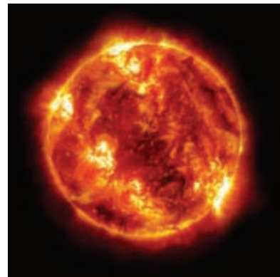
2.4 රූපය - සූර්යයා
